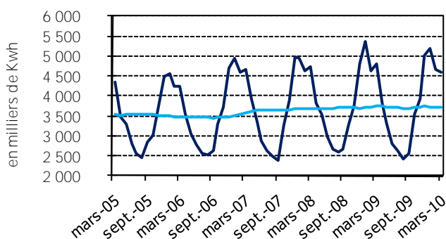
Electricité livrée au réseau
